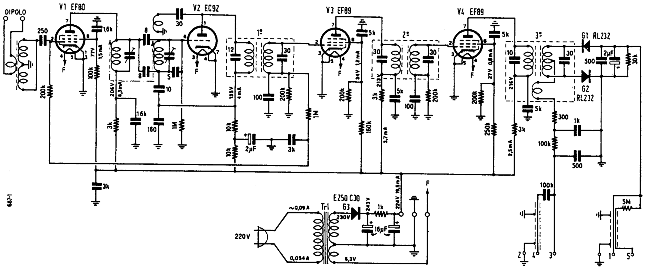
SCHEMA ELETTRICO DEL SINTONIZZATORE FM SABA-UKW-S5
